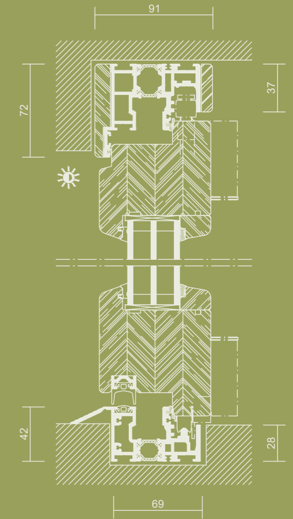
Vertikalschnitt | o.M.
